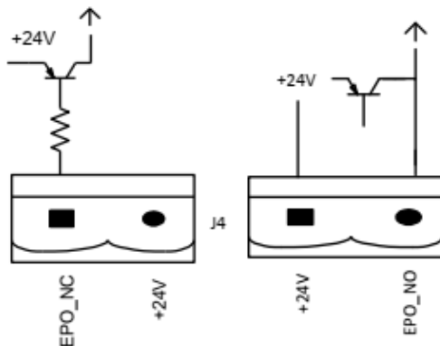
Рис. 2-16 Схема разъема системы экстренного отключения (ЕРО)
