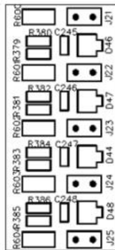
Рис.4-12 Расположение джамперов на главной плате управления (PS1203_CT1)
