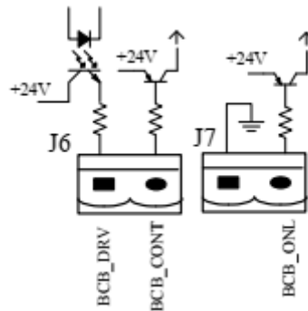
Рис. 2-18 Схема разъемов ВСВ
