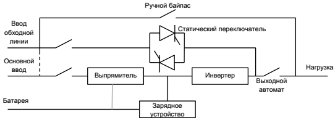
Рис.1-1 Схема ИБП
