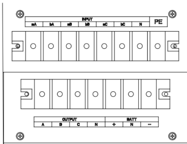
Рис. 2-13 Клеммная колодка на ИБП ЛЕГИОН-3Ф-40К-Ш
