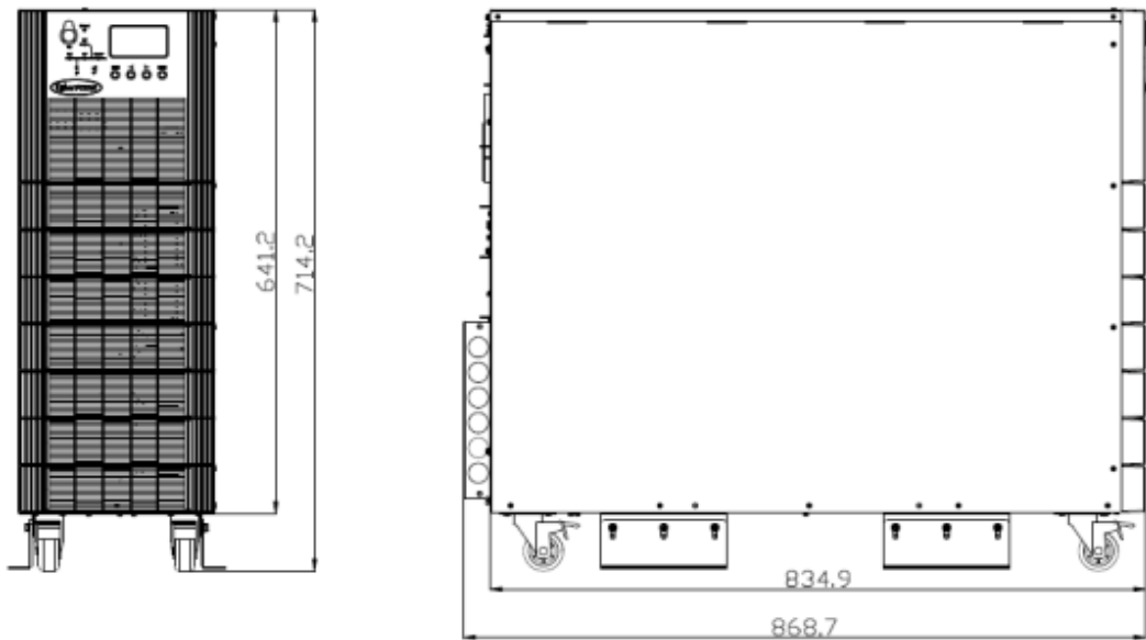
Рис.2-1-2 Габариты ИБП ЛЕГИОН-3Φ-10К-Ш (со встроенными батареями) (ед. изм.: мм)
