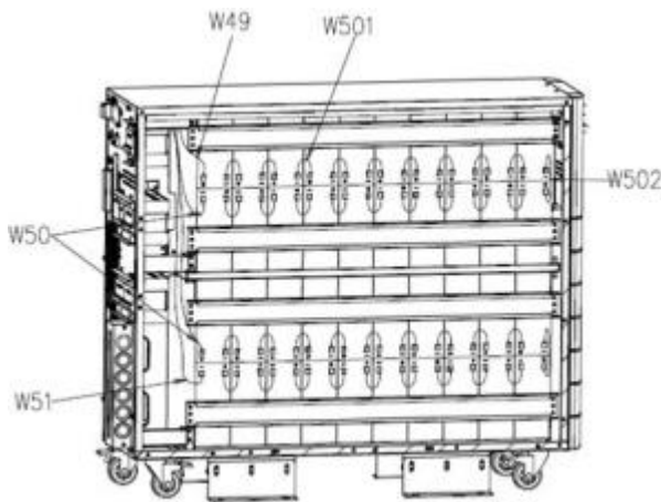
Рис.5-1 Установка батарей
