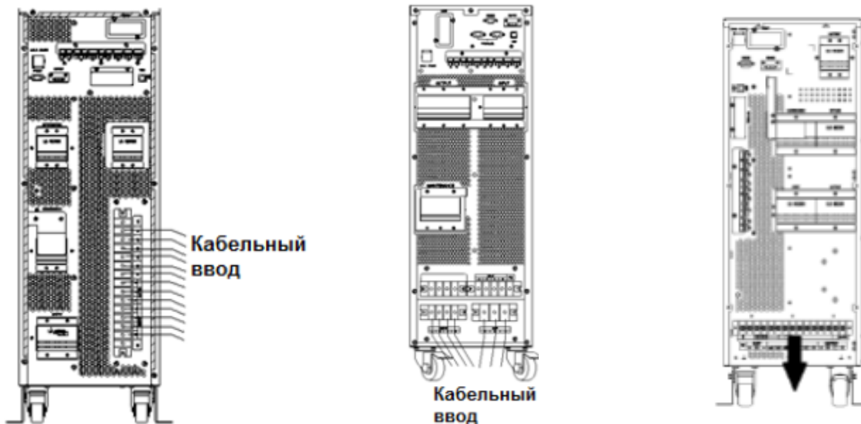
Рис. 2-10 Кабельный ввод
