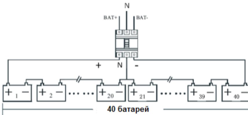
Рис. 2-9 Подключение батарей
