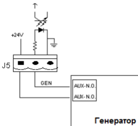
Рис. 2-17 Схема разъема «Работа с генератором»
