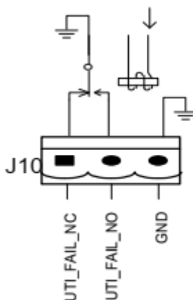
Рис.2-21 Схема разъема сигнала «Сбой электроснабжения»
