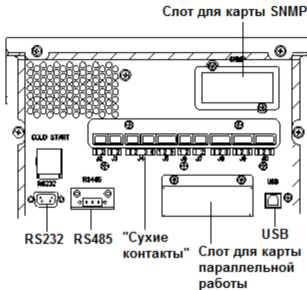
Рис.2-14 Коммуникационные интерфейсы
