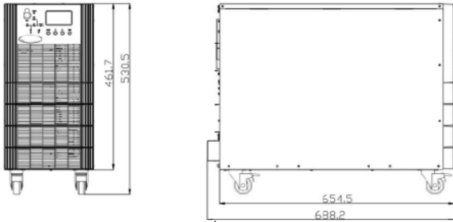
Рис.2-1-1 Габариты ИБП ЛЕГИОН-3Φ-10К-Ш/15-20К-С (без встроенных батарей) (ед. изм.: мм)
