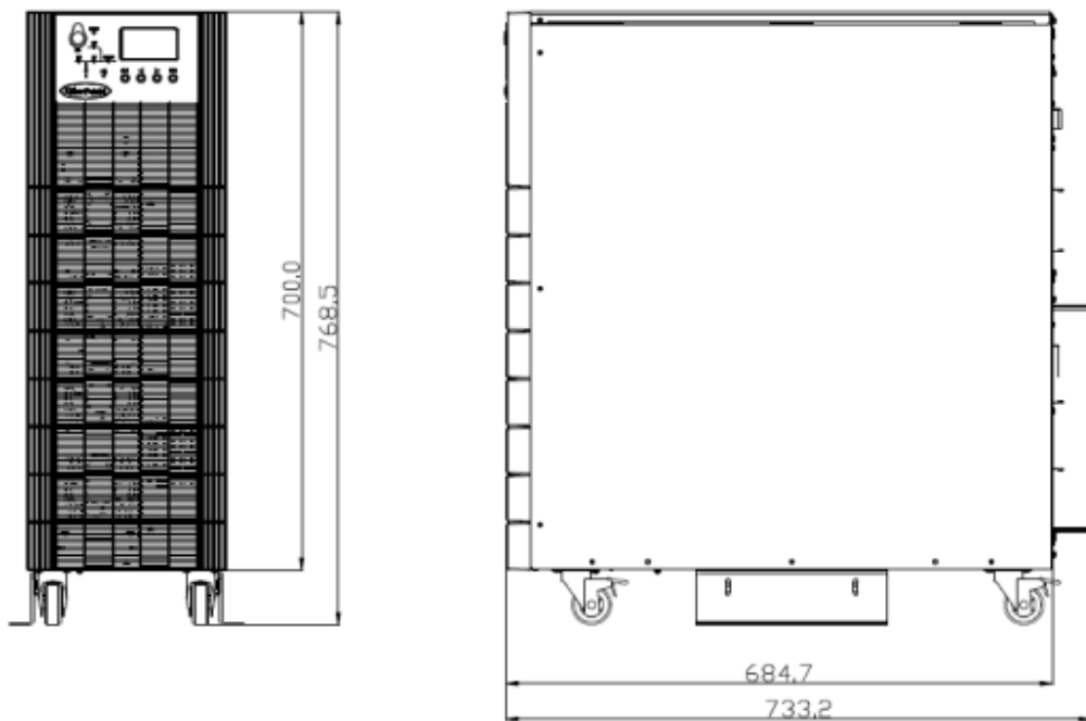
Рис.2-2-1 Габариты ЛЕГИОН-3Φ-20-30К-Ш/30-40К-С (без встроенных батарей) (ед. изм.: мм)
